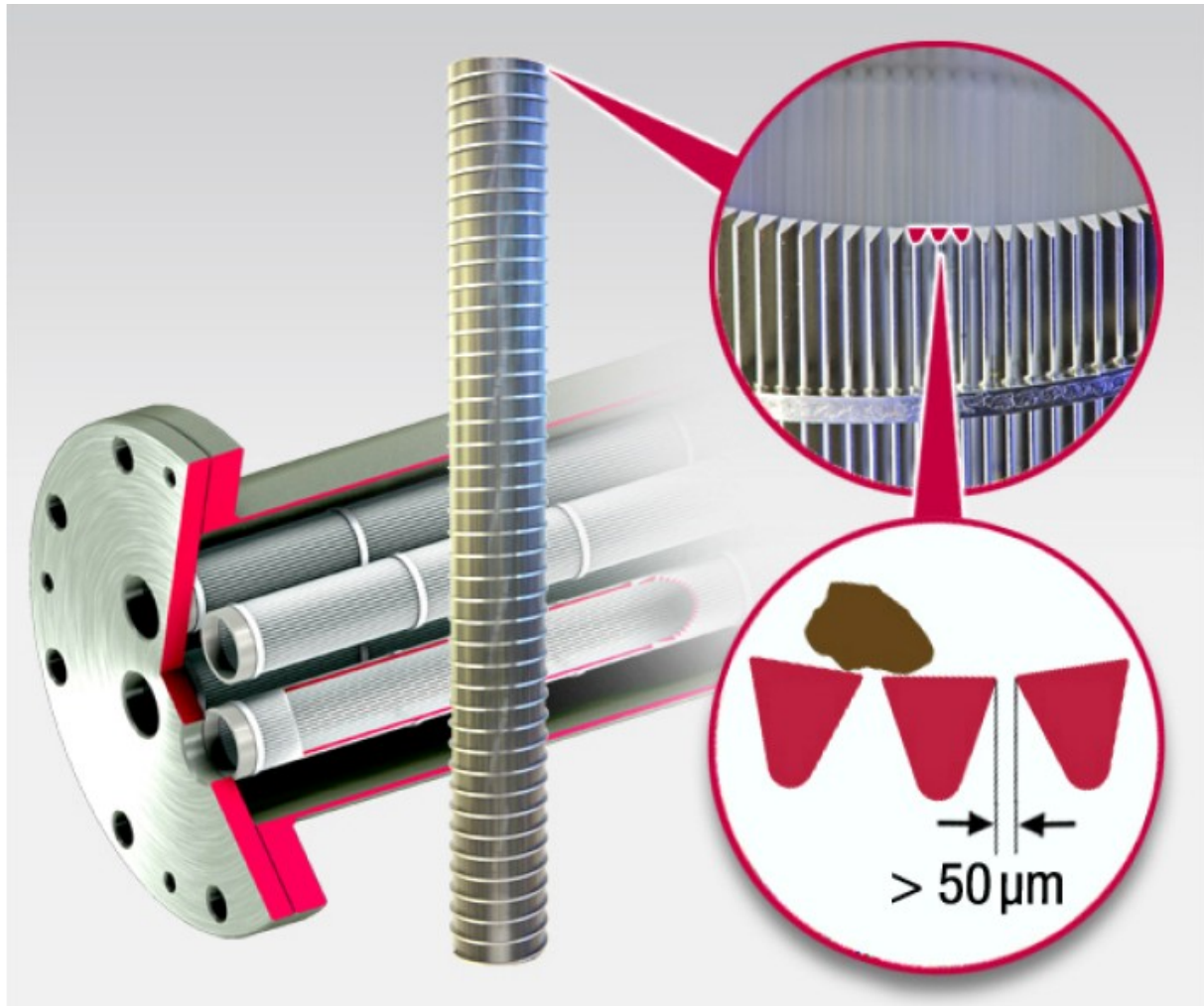
Filterstaver med langsgående spalteåpninger
